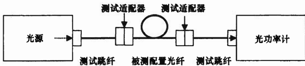
图 7 三跳线链路测试连接方式
