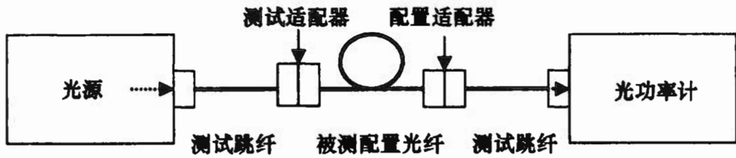
图 5 双跳线信道测试连接方式
