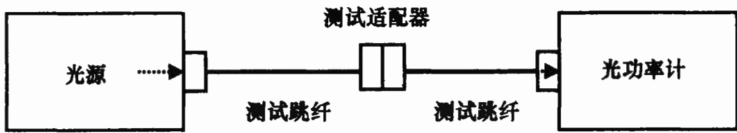
图 4 双跳线测试校准连接方式
