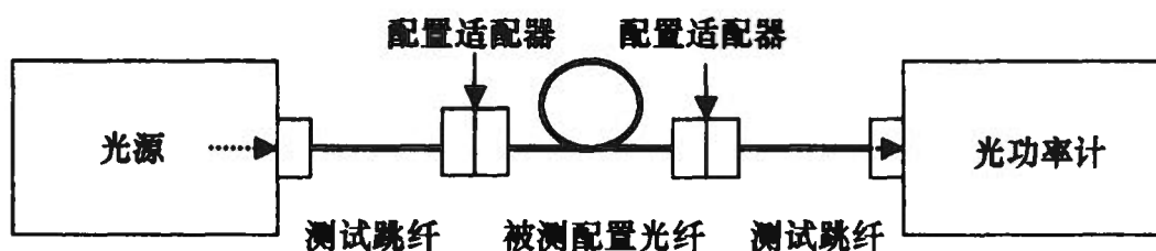
图 8 三跳线信道测试连接方式
