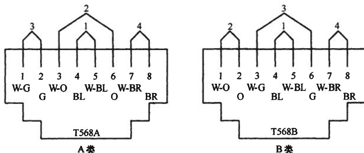
图 7.0.2-1 T568A 与 T568B 连接图
