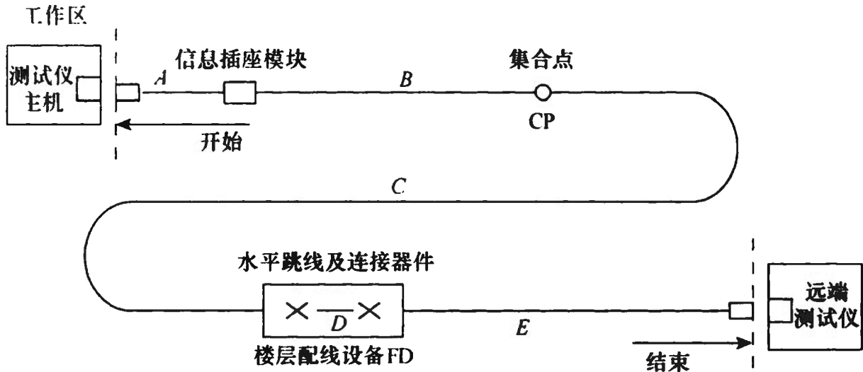
图 B.0.1-2 信道方式
