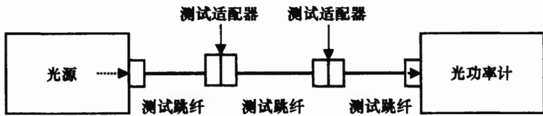
图 6 三跳线测试校准连接方式
