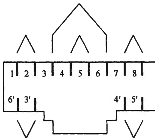
图 7.0.2-2 7 类和 7 A 类模块插座连接(正视)方式 1
