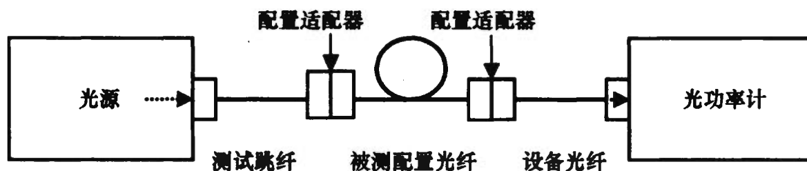
图 3 单跳线信道测试连接方式
