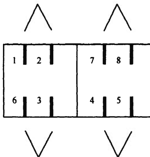
图 7.0.2-3 7 类和 7 A 类插座连接(正视)方式 2
