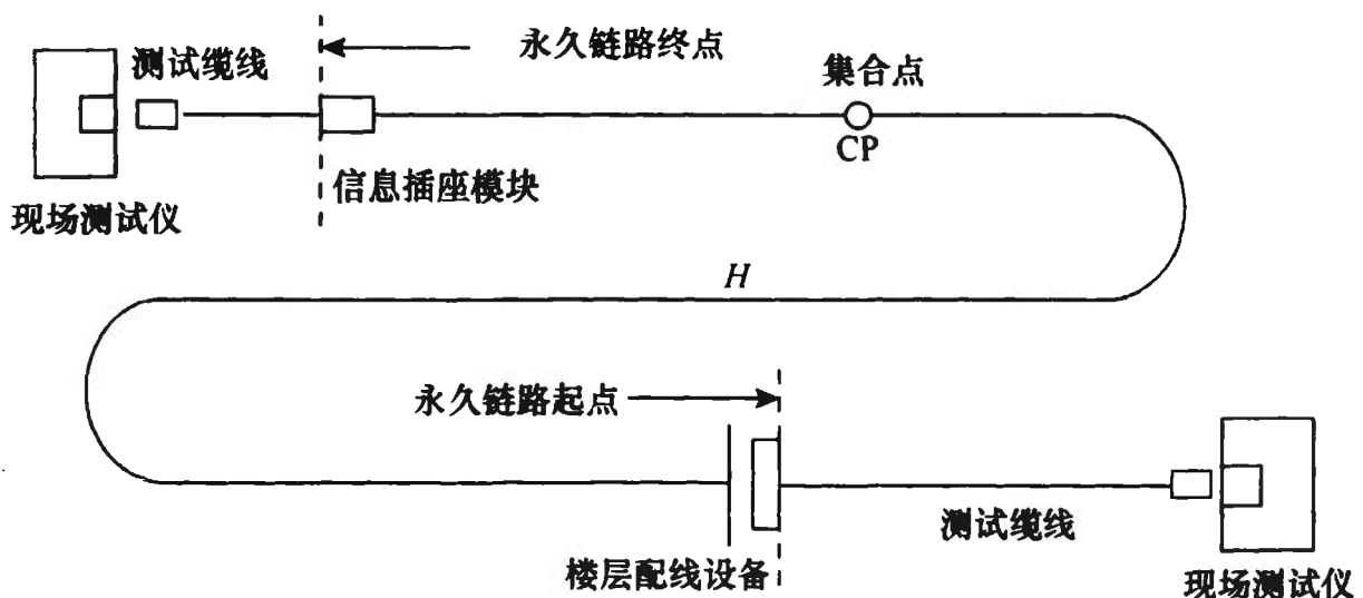
图 B.0.1-1 永久链路方式
